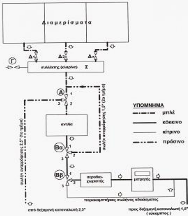
ΚΥΚΛΩΜΑ ΚΑΥΣΙΜΟΥ ΣΕ ΒΥΤΙΟΦΟΡΑ ΠΕΤΡΕΛΑΙΟΥ ΘΕΡΜΑΝΣΗΣ (Σε σύστημα αναρόφησης)
